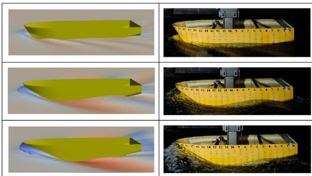
Patrón de olas numérico y experimental a diferentes velocidades.
