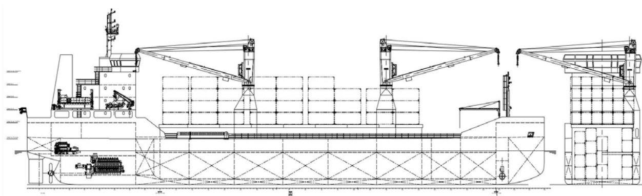
Plano general del buque a calcular.
