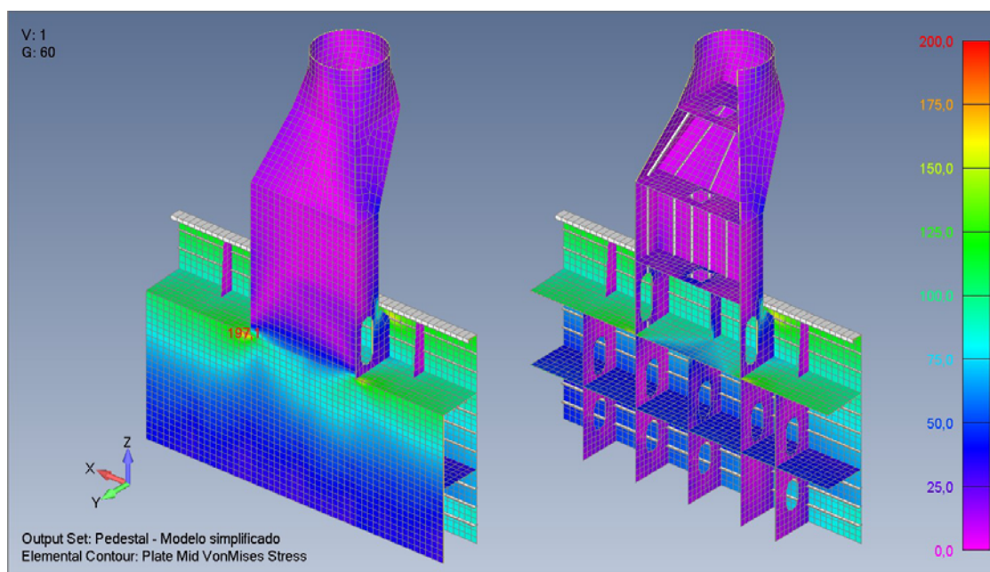
Resultado de medición de tensiones de VonMises al transportar contenedores, a fin de obtener indicadores de un buen diseño para materiales dúctiles.
