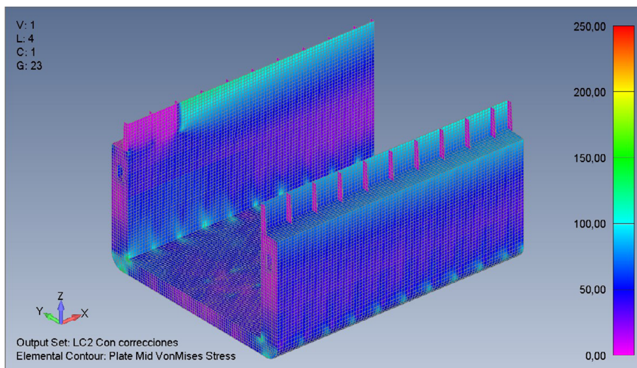
Análisis de tensiones en la bodega de carga.
